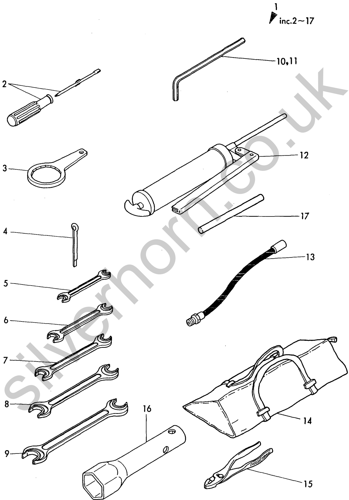
Fig. 4 コウグ(ゴムクローラ) TOOL (CRAWLER, RUBBER SPEC.)
