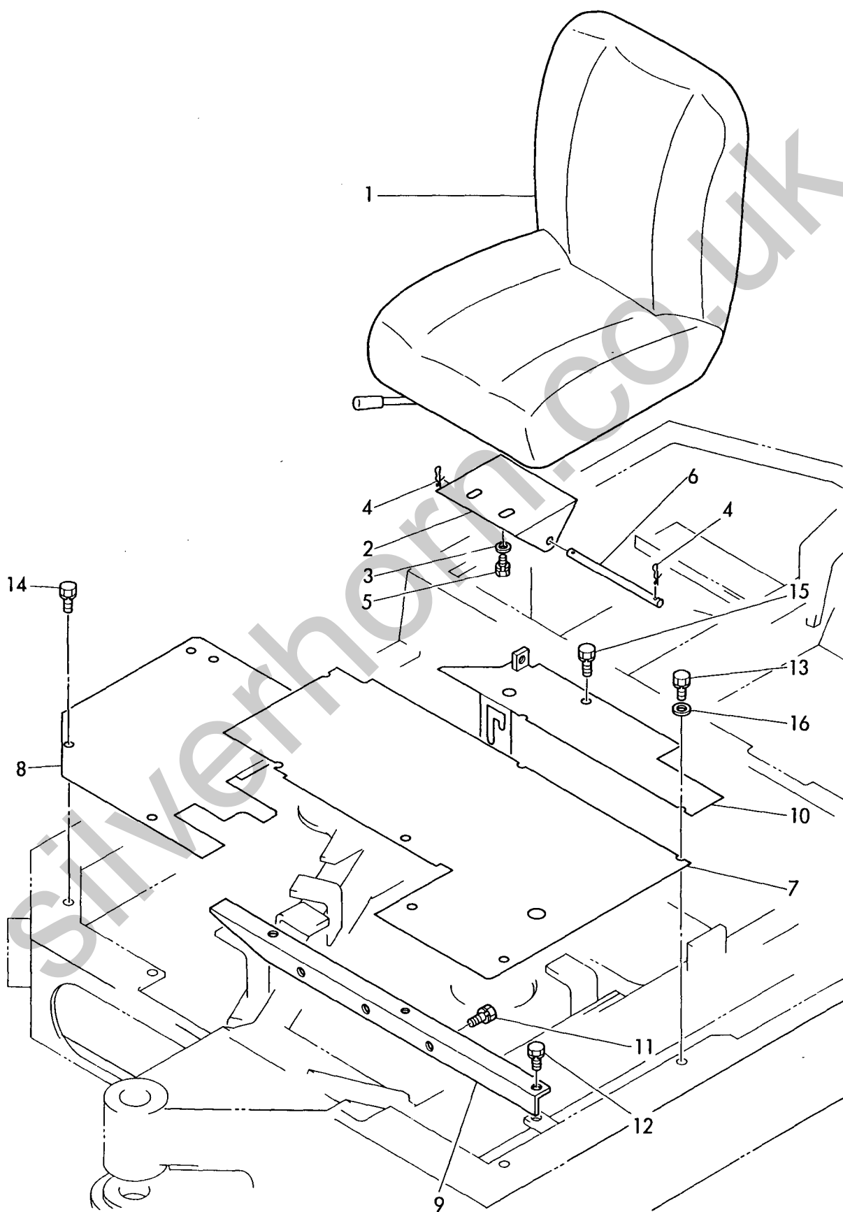
Fig. 27 シート & ステップ (キュウガタ) SEAT & STEP (PREVIOUS) (YB121U: M/ #00698マデ) (YB151U: M/ #00608マデ) (YB121U: TO M/ #00698) (YB151U: TO M/ #00608)
