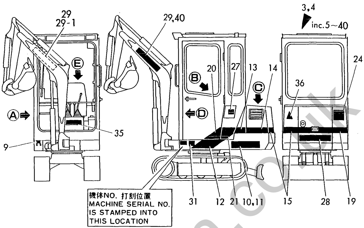
Fig. 2 メイバン(キャビン) LABEL (CABIN SPEC.)
