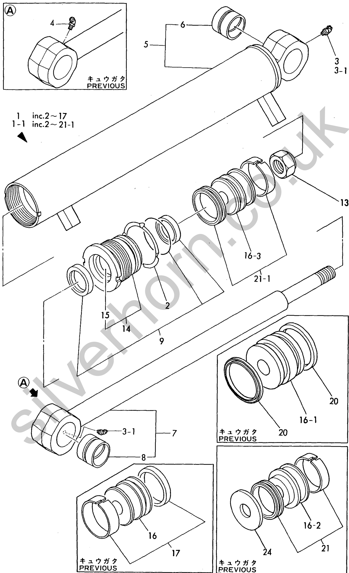
Fig. 53 アームシリンダ ARM CYLINDER
