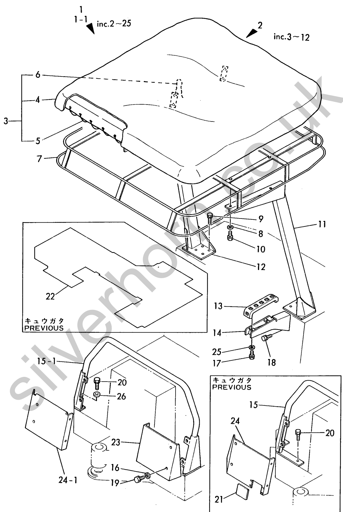
Fig. 29 キャンピ CANOPY
