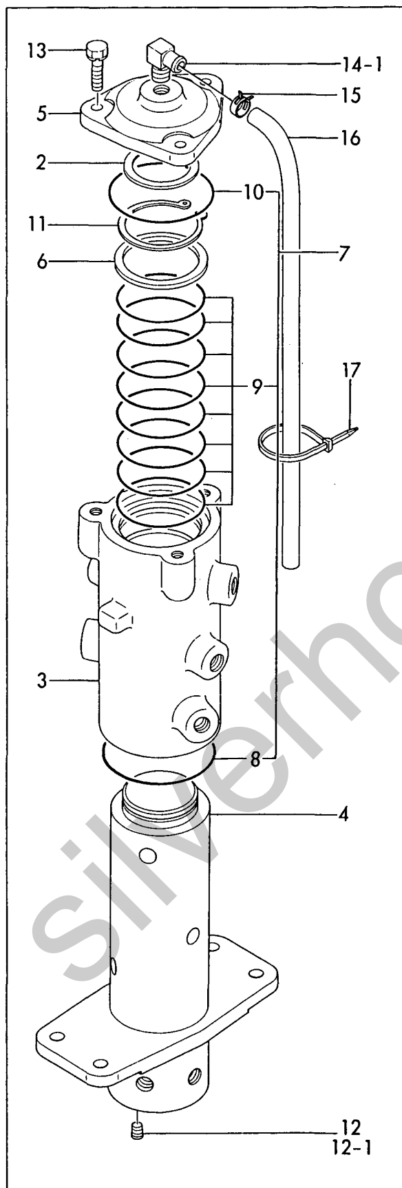
Fig. 57 スイベルジョイント SWIVEL JOINT
