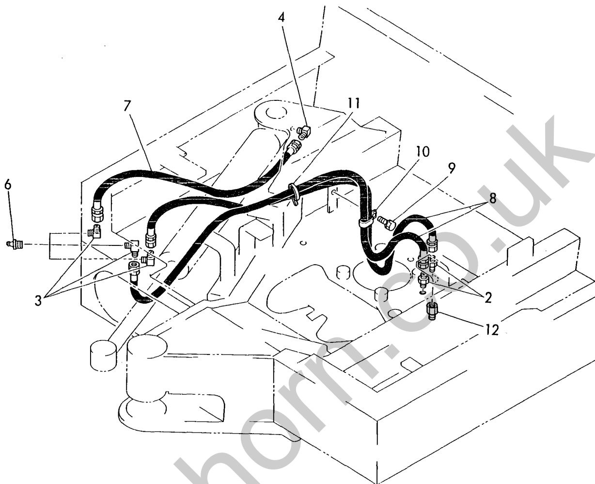
Fig. 33 エンカクキュウシ GREASING
