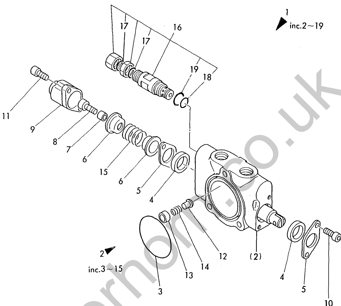
Fig. 49 コントロールバルブ(バケット) CONTROL VALVE (BUCKET)
