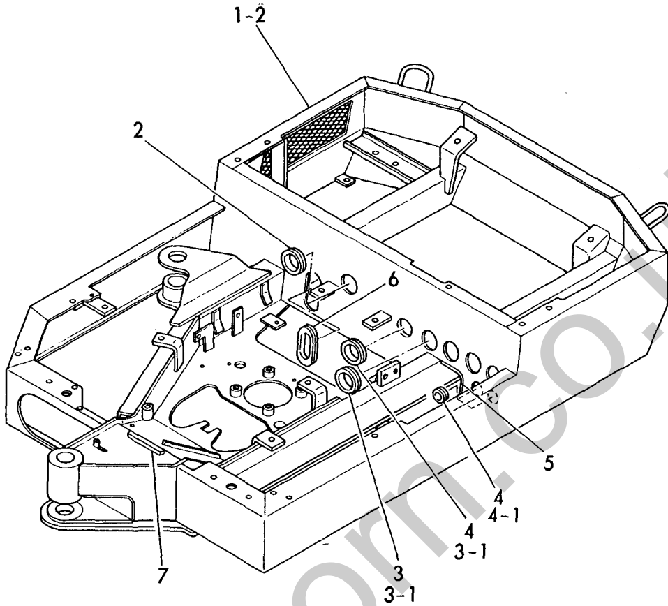
Fig. 22 センカイフレーム(YB121U) TURNING FRAME (YB121U)
