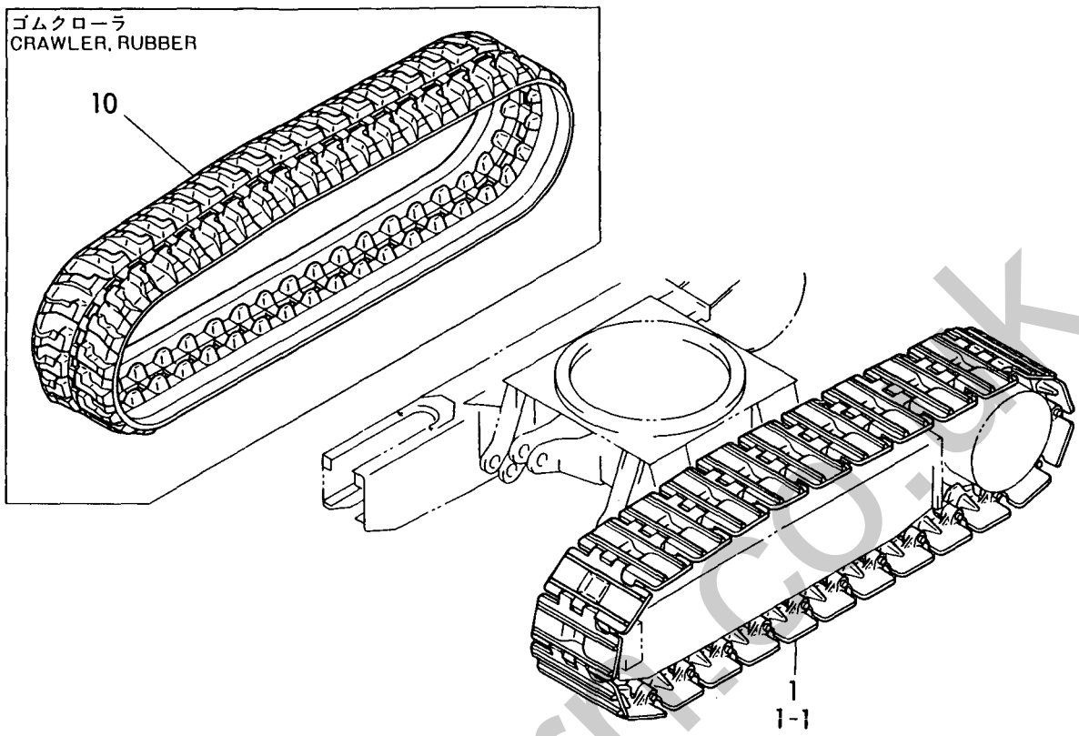
Fig. 17 クローラ CRAWLER
