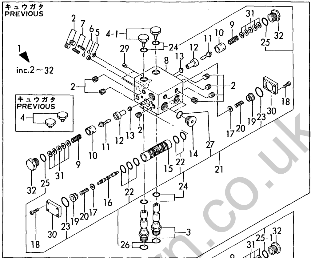
Fig. 59 ブレーキバルブ BRAKE VALVE
