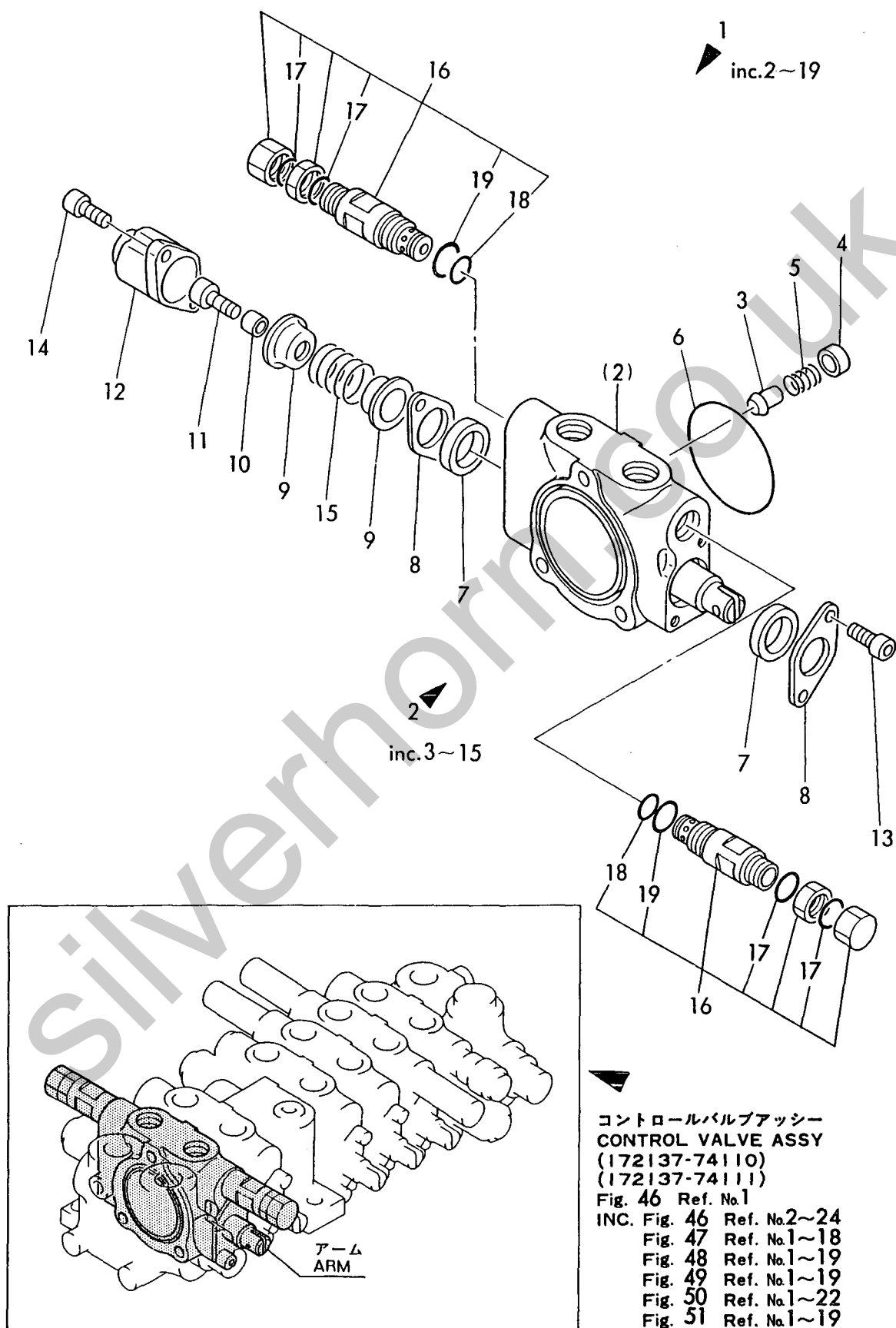
Fig. 51 コントロールバルブ(アーム) CONTROL VALVE (ARM)
