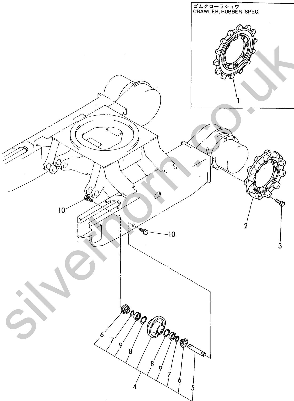
Fig. 15 トラックローラ TRACK ROLLER
