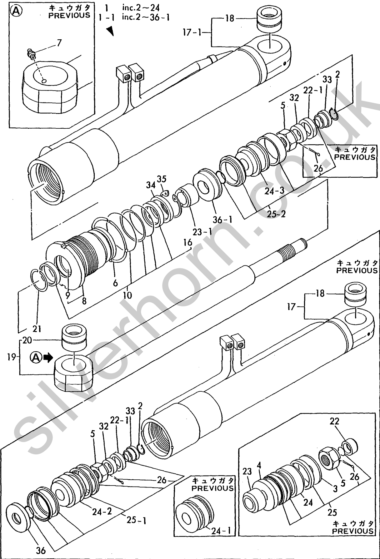
Fig. 55 スイングシリンダ SWING CYLINDER
