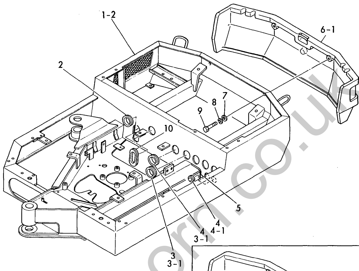
Fig. 23 センカイフレーム (YB151U) TURNING FRAME (YB151U)
