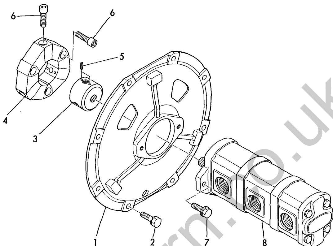
Fig. 32 ポンプ&ジクツギテ HYD. OIL PUMP & JOINT
