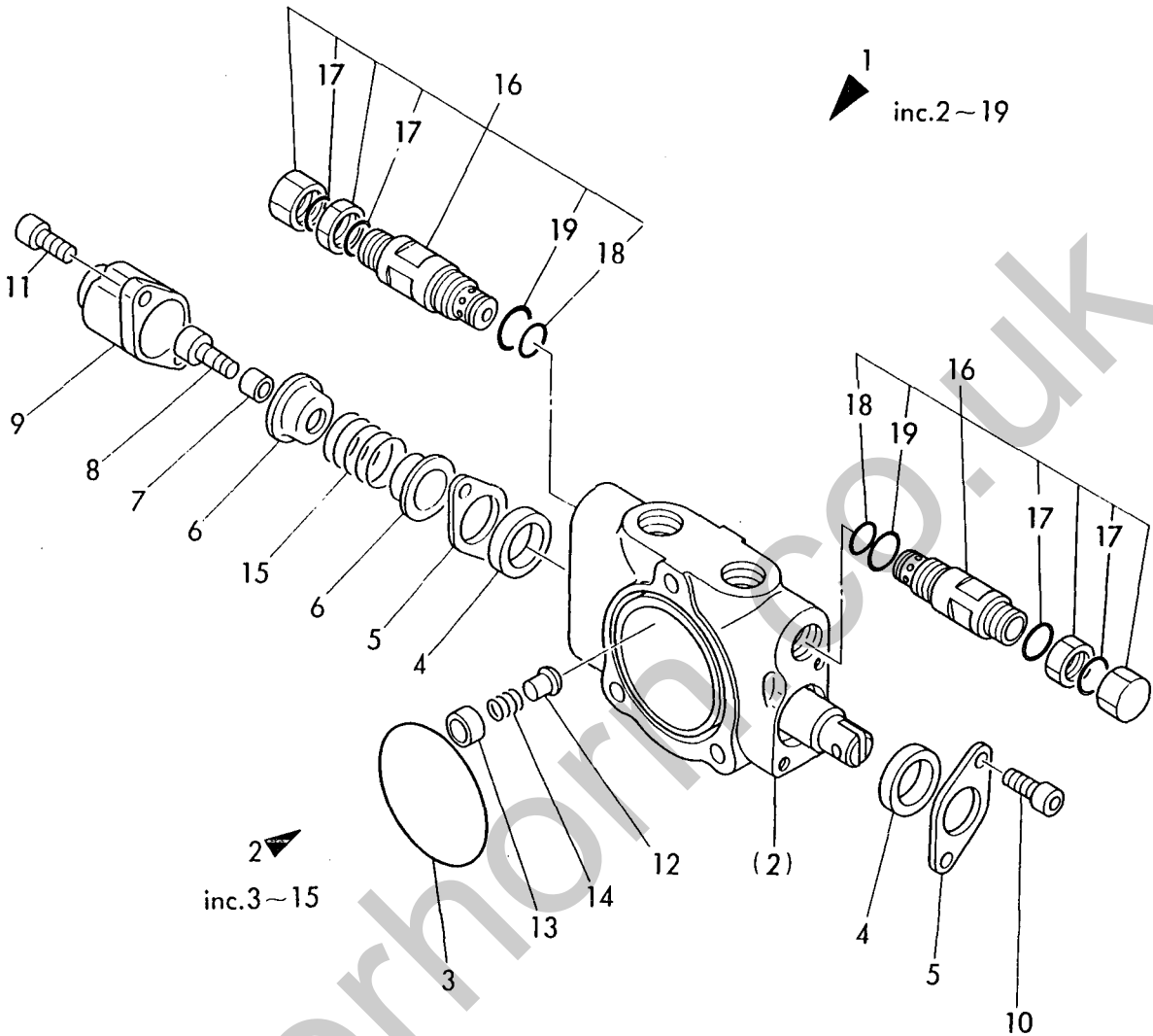
Fig. 48 コントロールバルブ(ブーム) CONTROL VALVE (BOOM)
